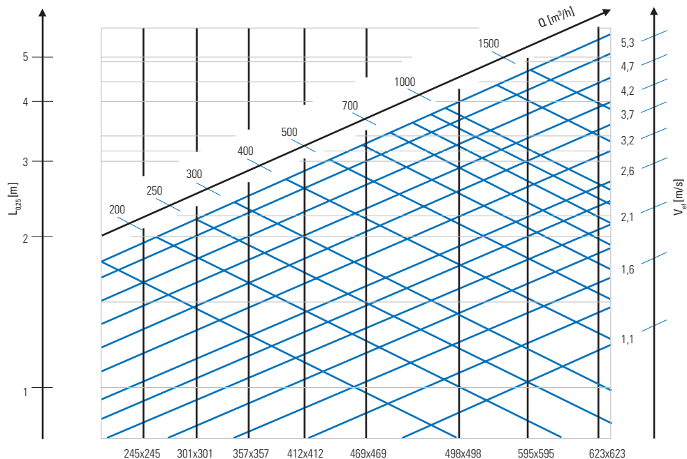
Anemostat ASW-3
