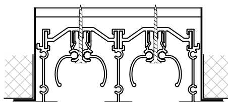
TYP C: mocowanie w ramie montażowej - blachowkręt zamocowany we wsporniku.
