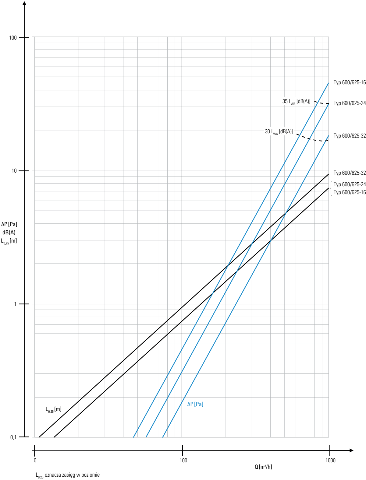
Diagram doboru dla nawiewników promieniowych AWR-3-1-PK i AWR-3-2-PK (kierownice ustawione pod kątem 45°)
