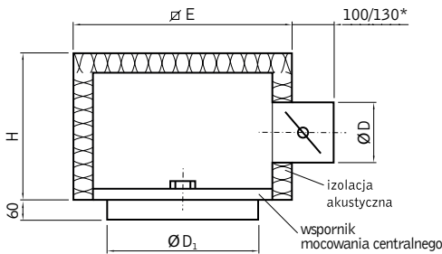
Standardowe wymiary skrzynek do nawiewników wirowych AWR-2
